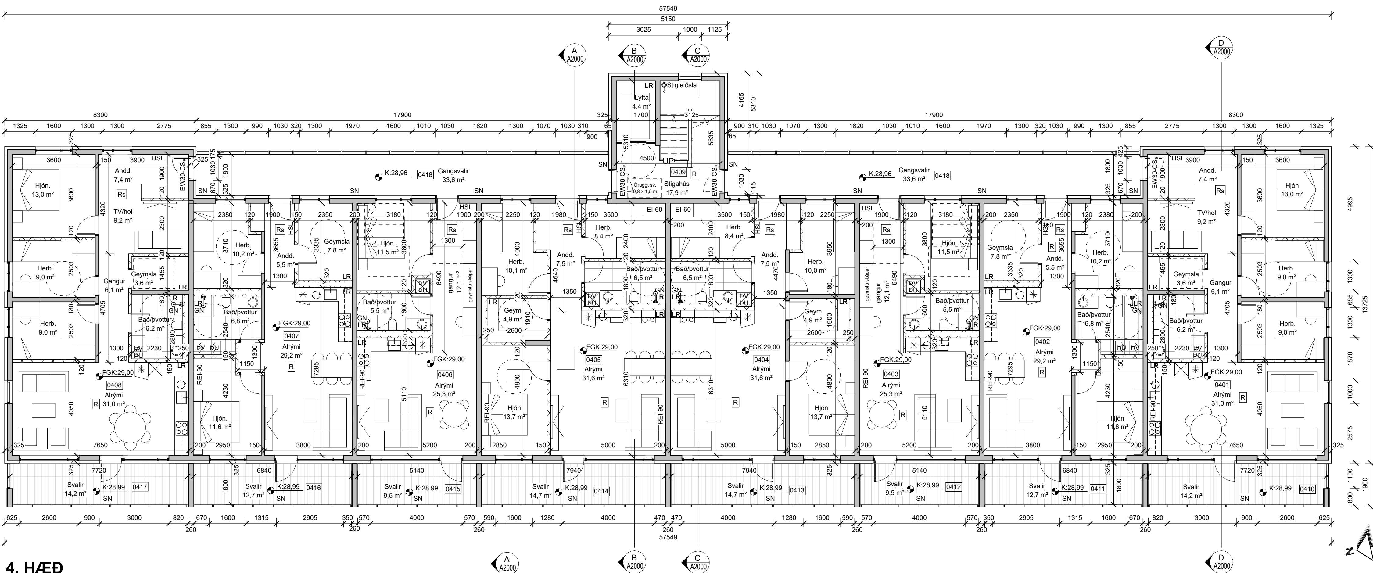
4. HÆÐ mkv: 1 : 100
