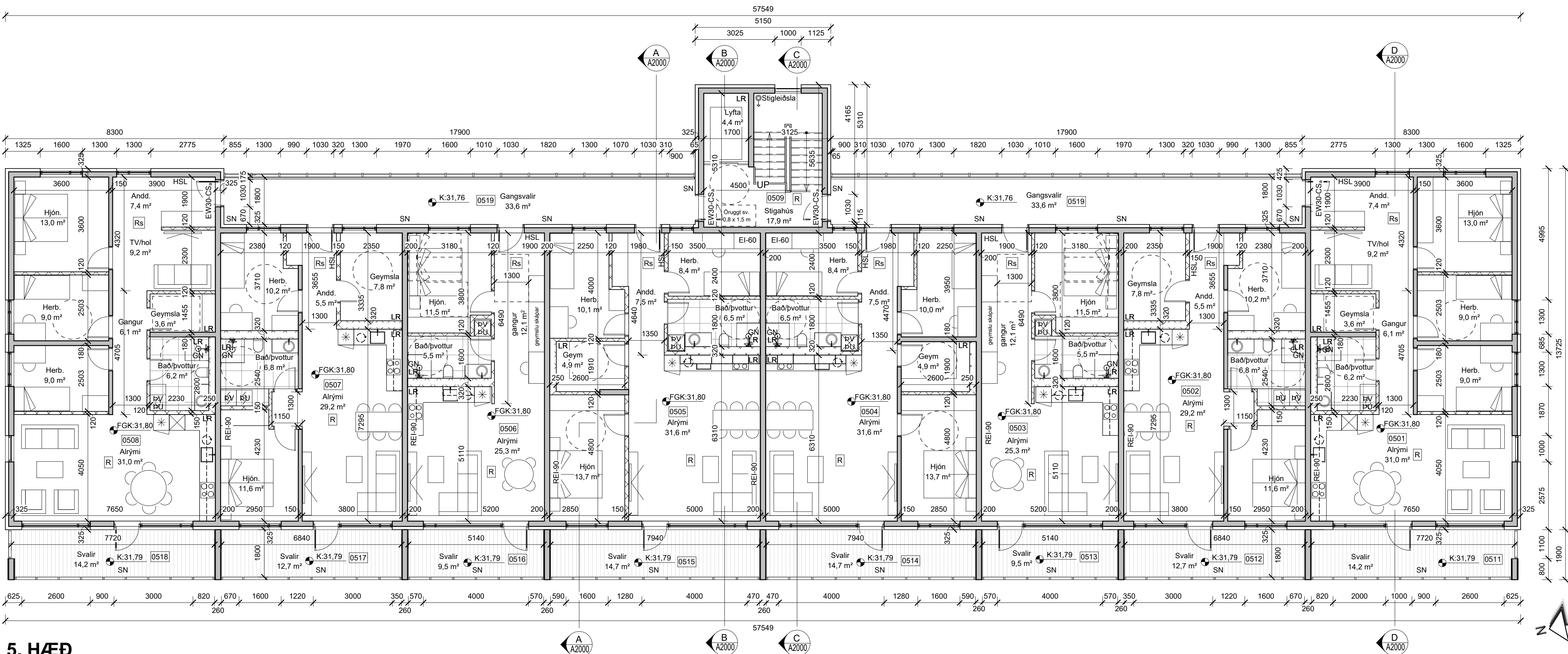
5. HÆÐ mkv: 1 : 100
